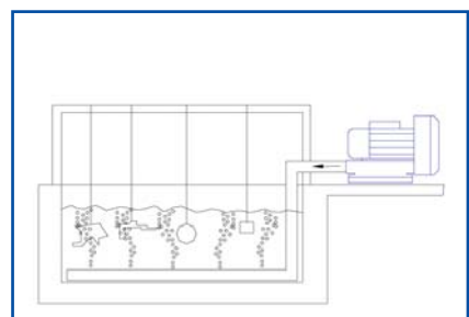
Baños electrolíticos Electrolyte Stirrer
