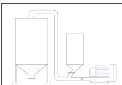
Transporte Neumático Powder & Granule Conveyor
